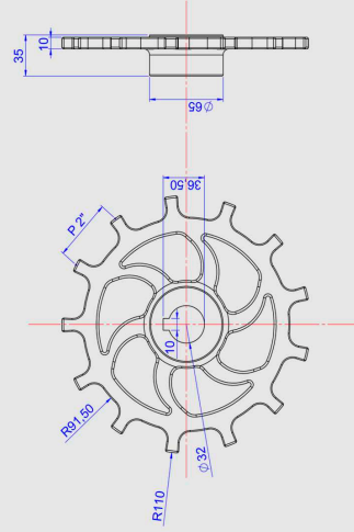
Engrenagem Guia/Motriz p/Esteiras 220 x 32mm Z13 (P. 2") Material: CF-8 (Aço Inox 304)
