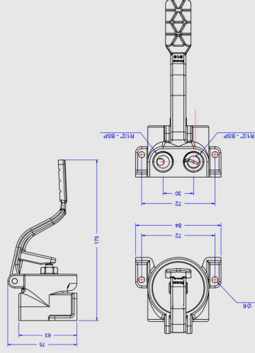
Válvula de Acionamento Pedal E-1/2"BSP (Interna) X S-1/2"BSP (Interna) Material: CF-8 (Aço Inox 304)
