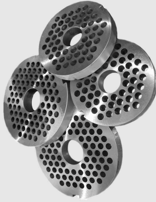
Discos P/ Moedores Diversos Material: Aço IC 4340
