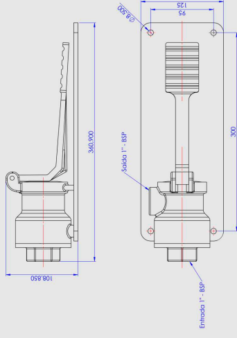
Válvula de Acionamento Pedal 3 Estágios E-1"BSP (Interna) X S-1"BSP (Interna) Material: CF-8 (Aço Inox 304)
