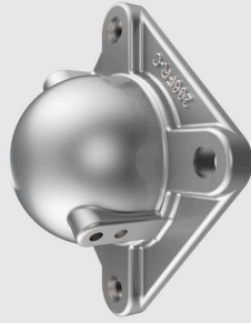
Mancal FR-C (Flange 4 Furos) 206FR-C (Cego) Material: CF-8 (Aço Inox 304)
