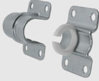
Mancal Intermediário do Varão ø25mm Material: CF-8 (Aço Inox 304)
