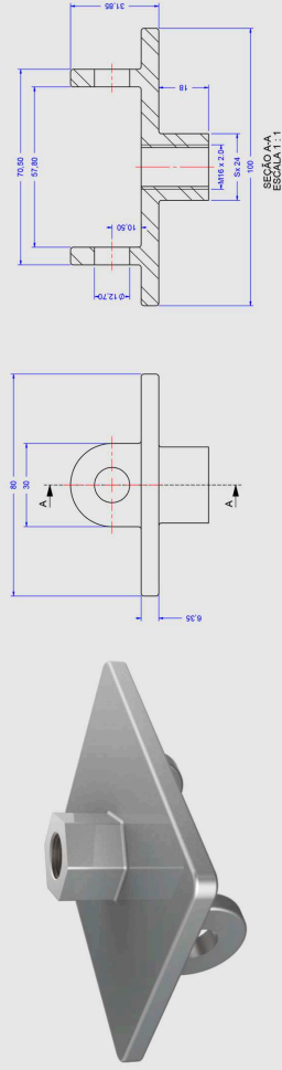
Base do Cone p/ Esteira de Cortes Material: CF-8 (Aço Inox 304)
